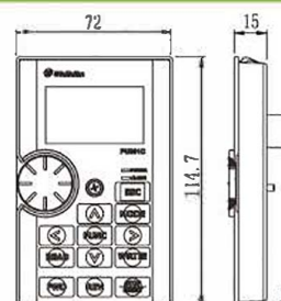
PU301C 尺寸圖
