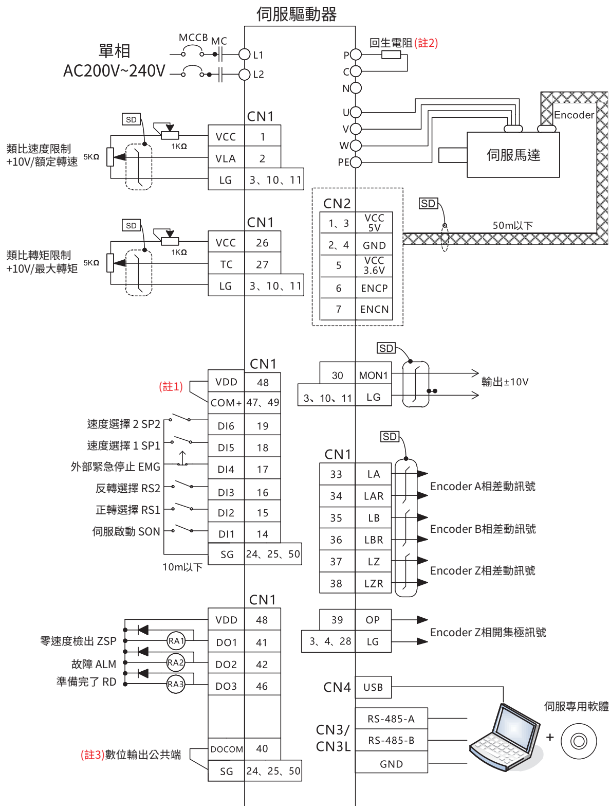
T Mode: 扭力控制模式接線示意圖
