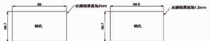
〈卡扣安裝面板開孔尺寸圖〉
