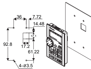
盤面安裝開孔尺寸圖
