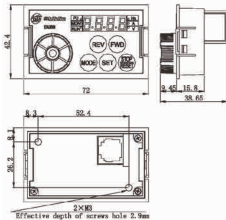
DU06尺寸圖
