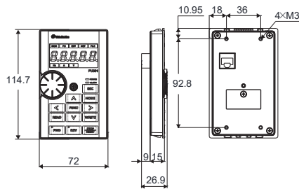
外型尺寸圖
