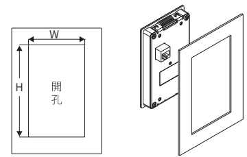
卡扣安裝開孔尺寸圖
