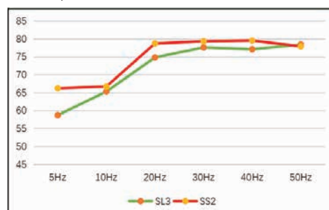
雜訊對比(db) 與舊產品相比, 低頻雜訊明顯改善
