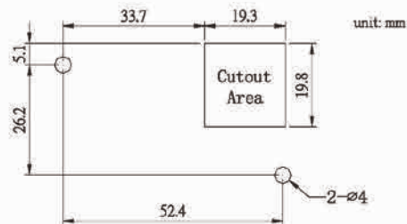
卡扣安裝面板開孔尺寸圖，鋼板厚度建議為2mm
